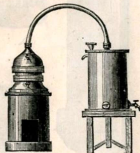
Petits alambics d'essai avec fourneau et trépied.
