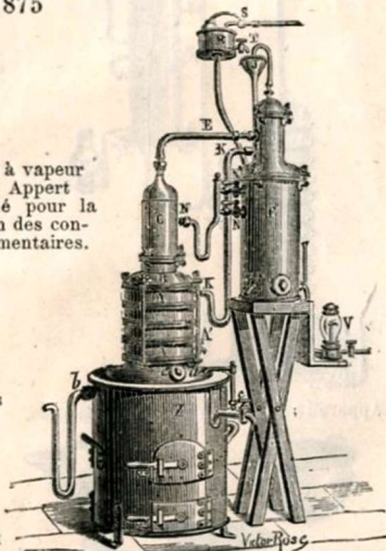
Appareil ÉGROT, petit modèle, vendu avec fourneau et trépied.
